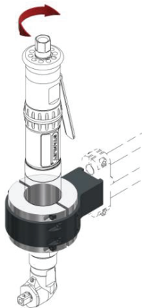
VERTICAL ROTATION CLAMP P/N: 100119
