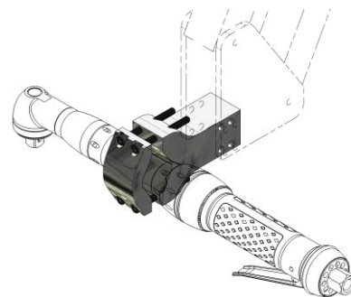
HORIZONTAL V-BLOCK P/N: 658532
